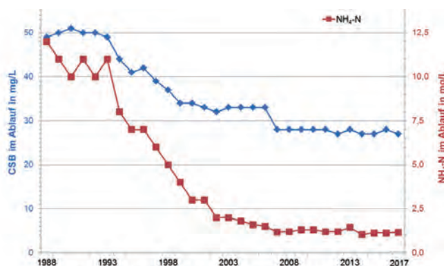
CSB und NH 4 -N-Ablaufwerte
