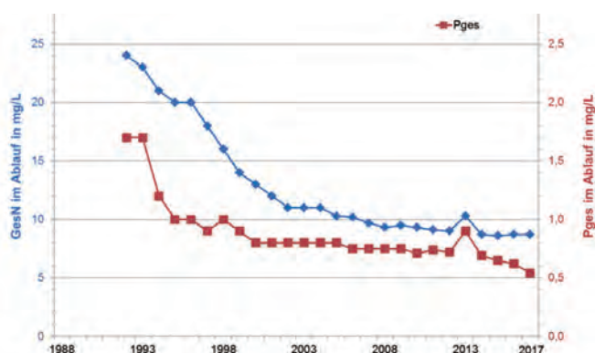
GesN und Pges-Ablaufwerte
